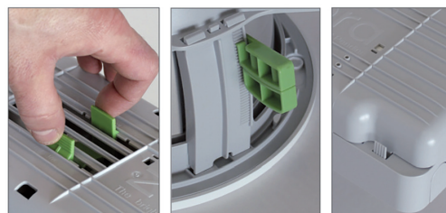
Justering av ljuskälla
